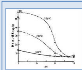
マグネタイトの溶解度とpH
