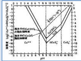
銅成分の溶解度とpH
